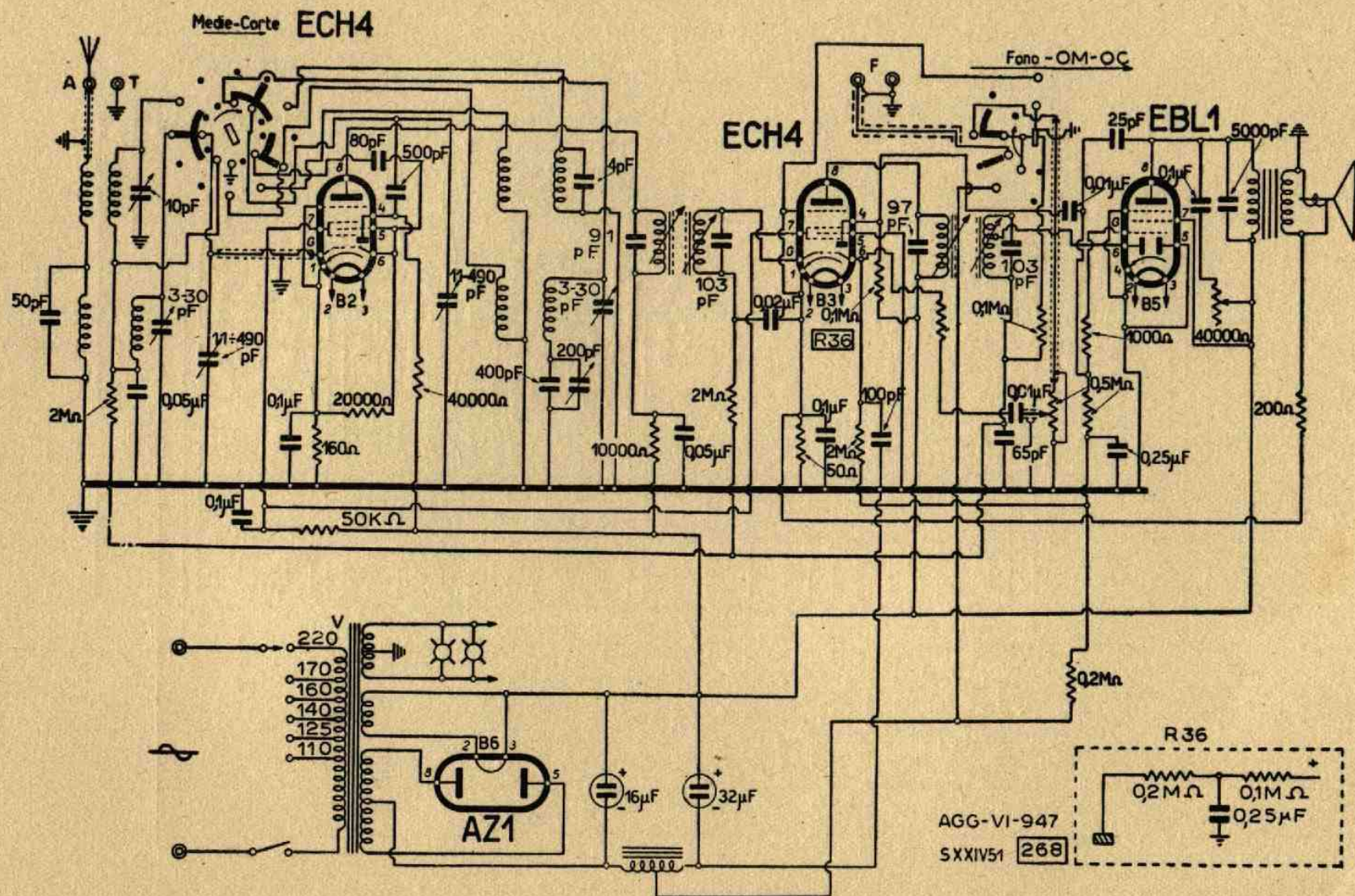
Lo schema elettrico dei modd. BI 460/A - BI 471/A - HI 470 A.
